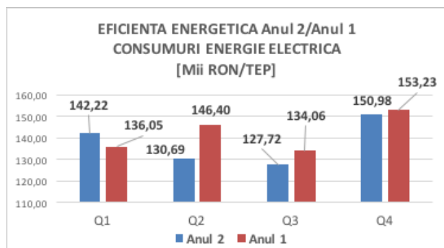
Fig. 16 Eficiența energetică trimestrială a consumurilor de energie
