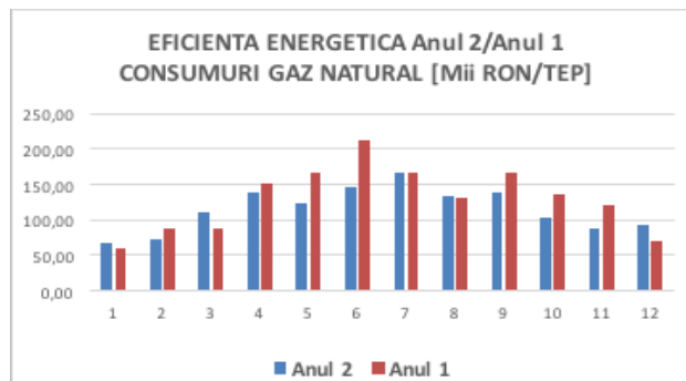
Fig. 15. Eficiența energetică lunară a consumurilor de energie
