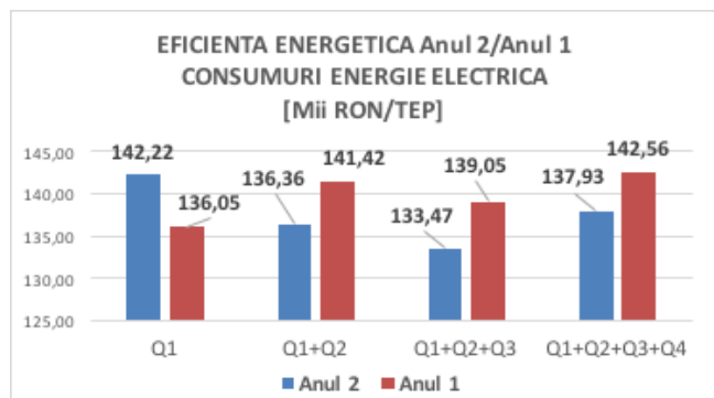
Fig. 17. Eficiența energetică anuală a consumurilor de energie
