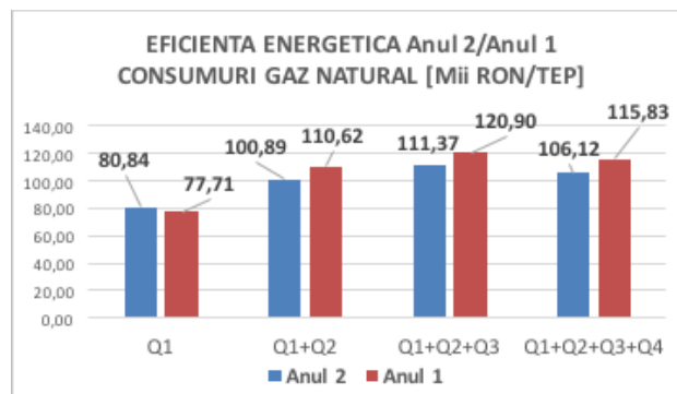
Fig. 17. Eficiența energetică anuală a consumurilor de energie
