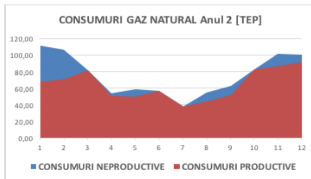
Fig. 5. Consumuri de gaz natural Anul 2/Anul 1
