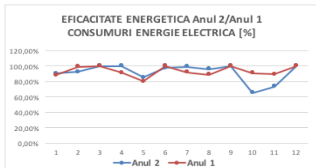
Fig. 18. Evoluția eficacității energetice
