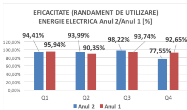
Fig. 20. Eficacitatea trimestrială a consumurilor de energie
