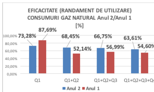
Fig. 21 . Eficacitatea energetică anuală a consumurilor de energie
